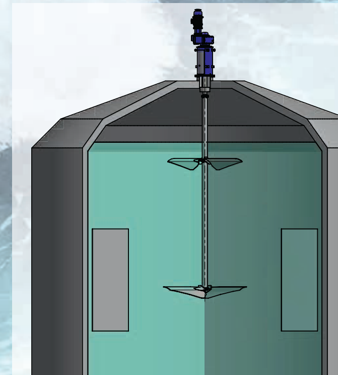
Faulraumrührwerk mit einer Wellenlänge von 20 m
